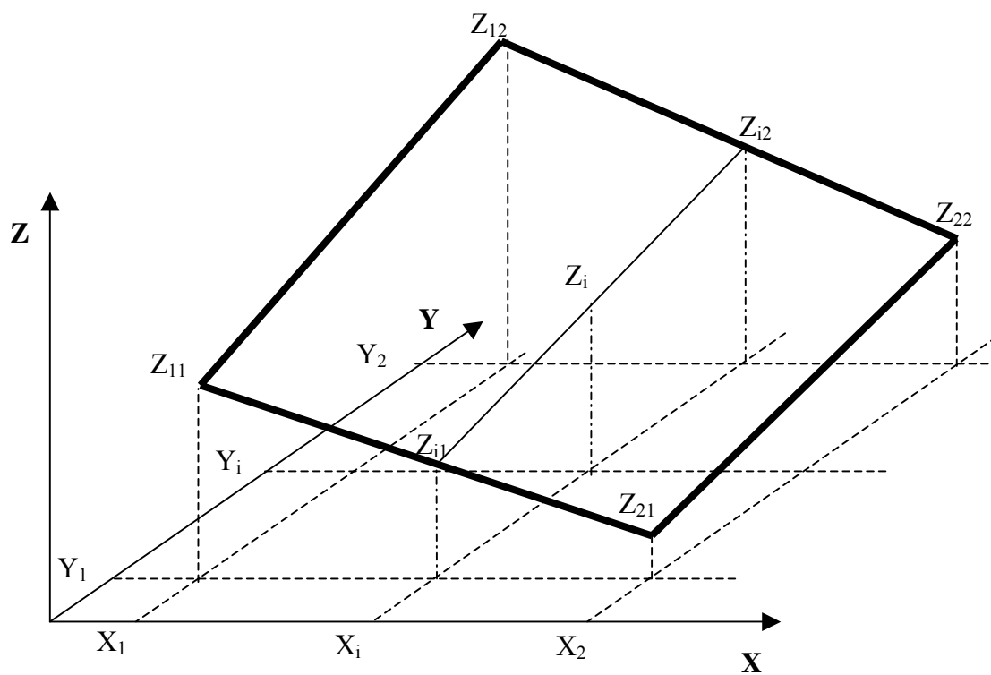
Рис. 3. Схема алгоритма линейной интерполяции:
