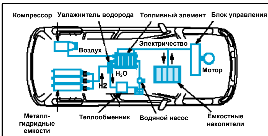
Рис. 31. Компоновочная схема электрокара на топливных элементах Mazda Demio FCEV
