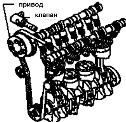
Рис. 22. Схема системы газораспределения с переменными фазами
