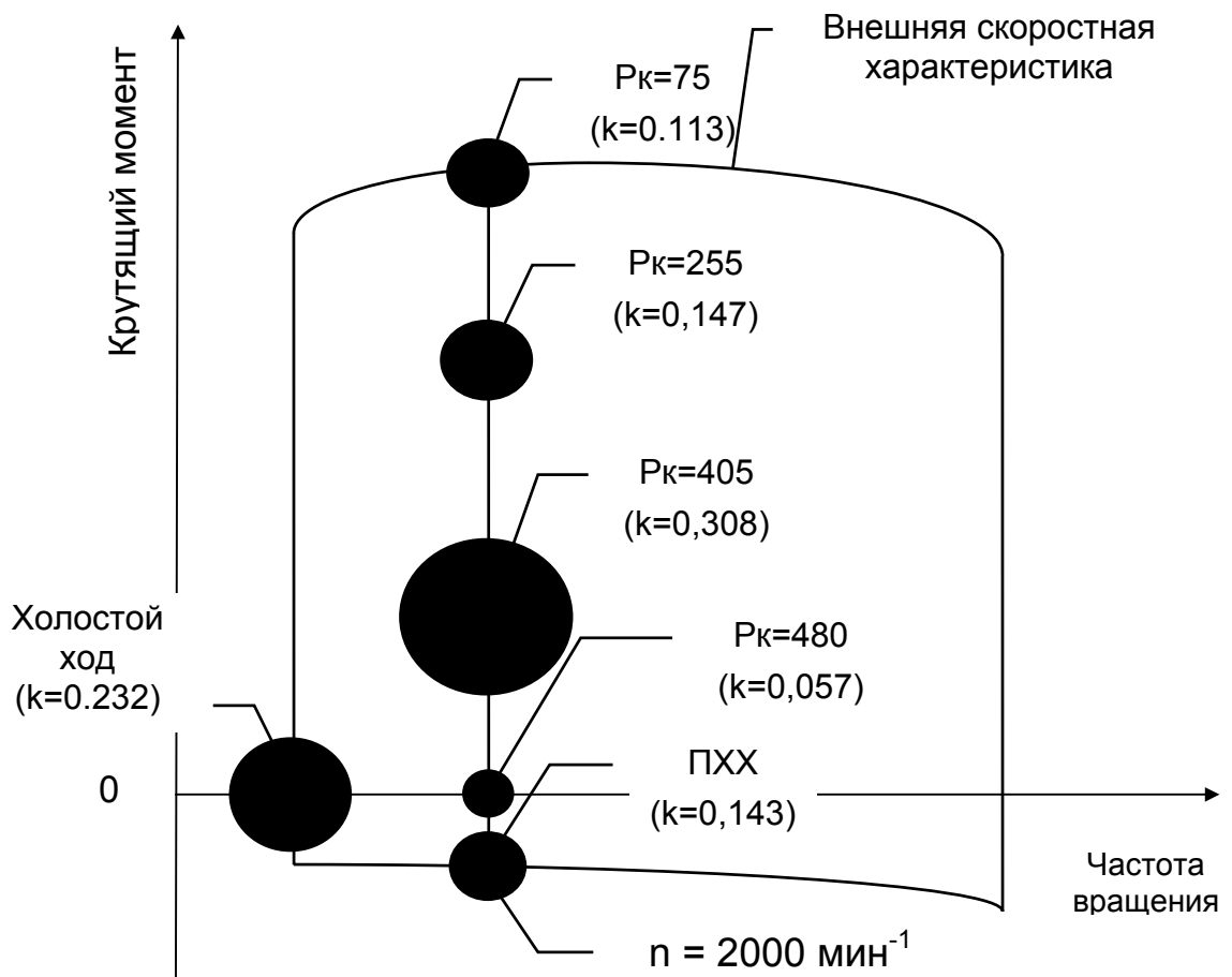
Рис. 6. Режимы испытаний двигателя по ОСТ 37.001.070-94
