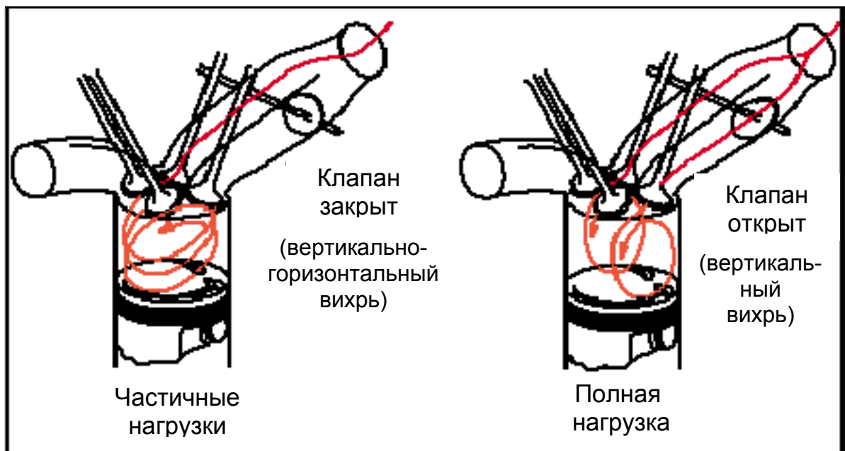
Рис. 19. Схема формирования вихря в двигателе, работающем на бедных смесях
