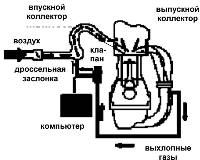
Рис. 21. Схема системы рециркуляции отработавших газов
